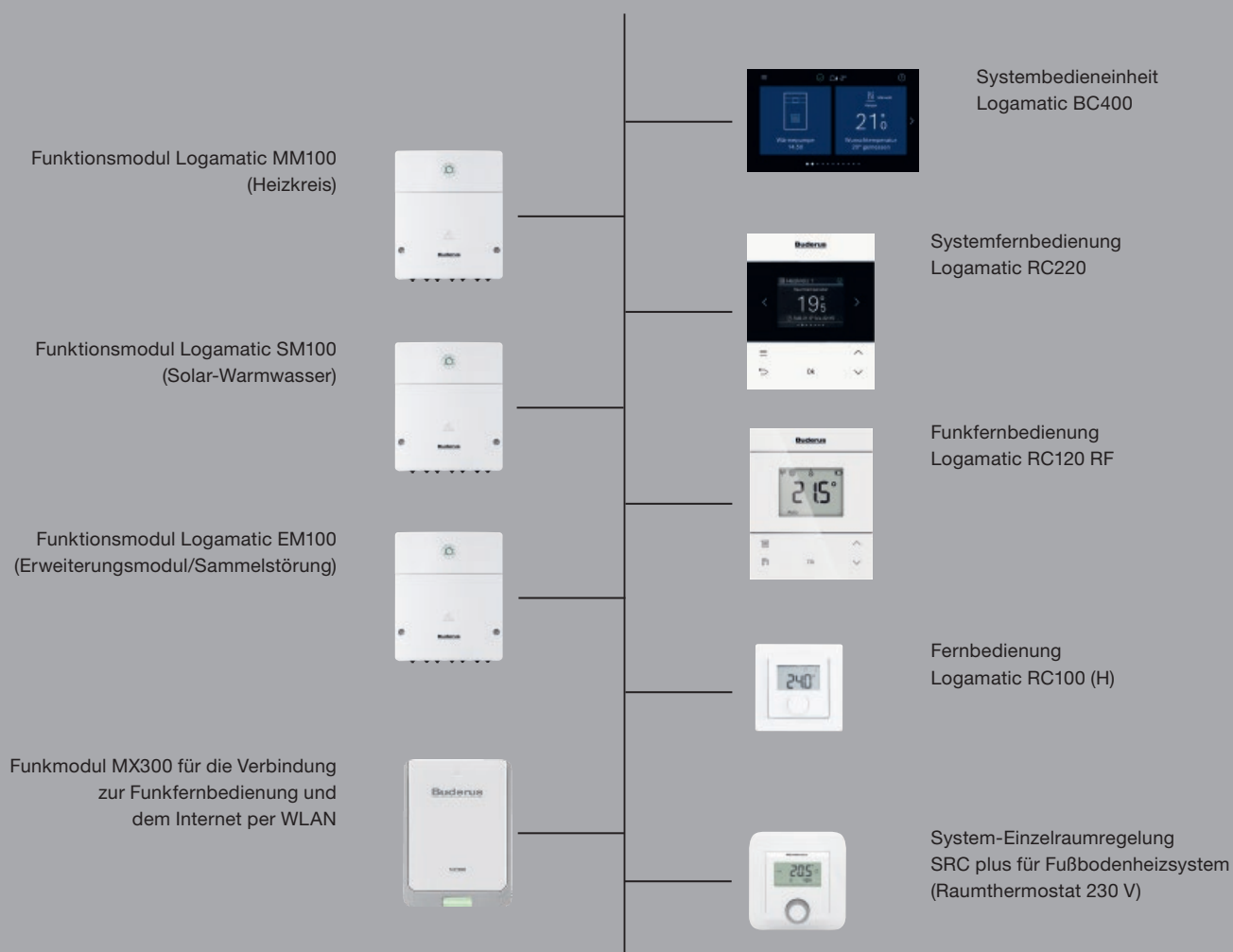
Wärmepumpe Logatherm WLW186i AR / WLW176i AR
